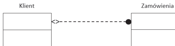
Rysunek 1.14. Diagram związków encji zapisany w różnych notacjach
